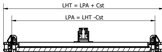
A-A ( 1:10 )
