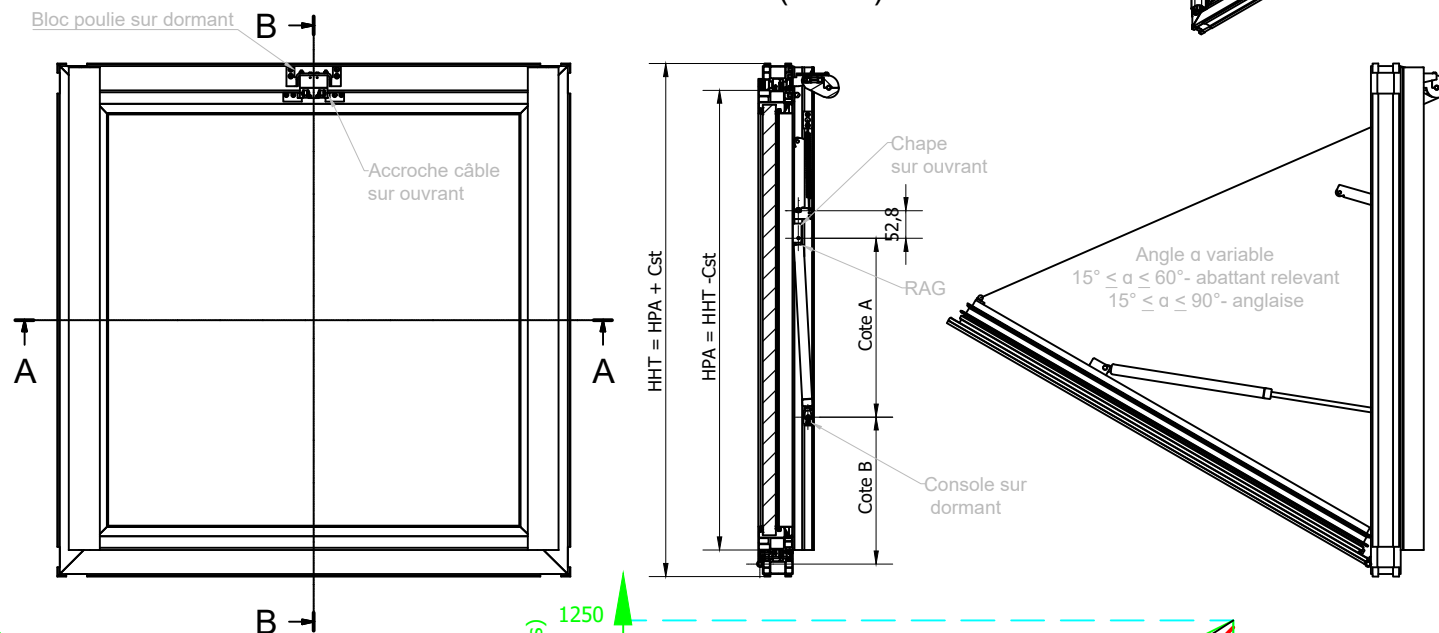
B-B ( 1:10 )
